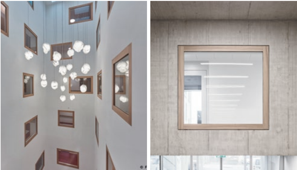
Festverglasungen in Lichthöfen sind essenziell , da sie die Ausbreitung von Feuer und Rauch effektiv verhindern. Gleichzeitig bewahren sie natürliches Licht in Gebäuden und sorgen für eine natürliche Atmosphäre. Je nach Anforderung können sie zudem erweiterten Schutz vor Einbrüchen, Lärmbelastung, Absturz und sogar Beschuss bieten.
